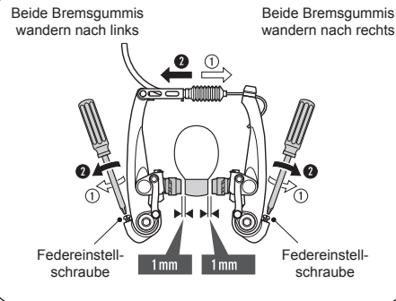
Einstellen der Bremsen an der Felge
